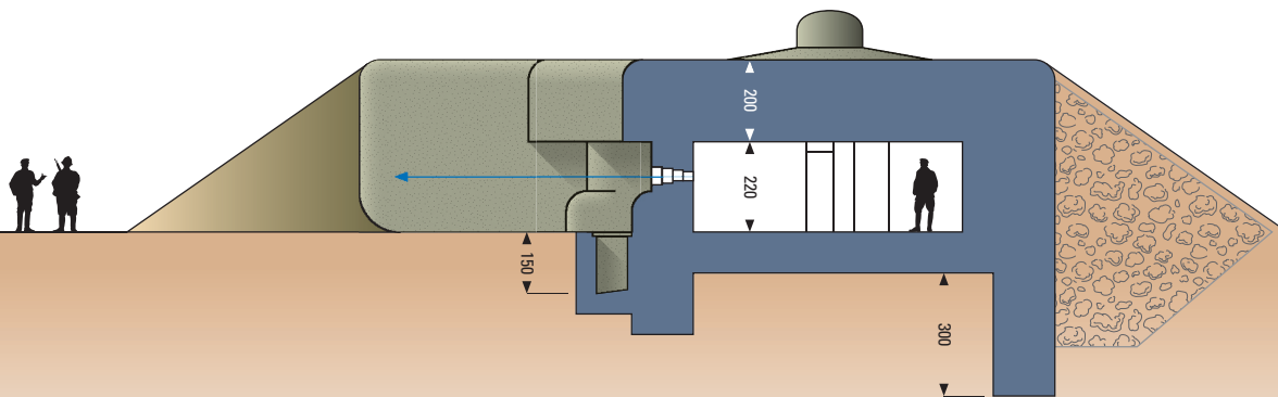
Coupe suivant A A'
